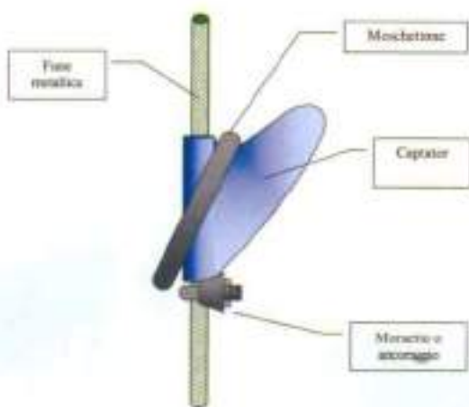
Fig. 7. Sopra: Captatore ad aletta
