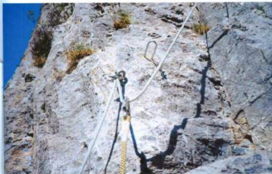
Qui sotto: L'ansa a fine corsa, suggerita da Baille e adottata nelle prescrizioni francesi (foto G. Bressani).
