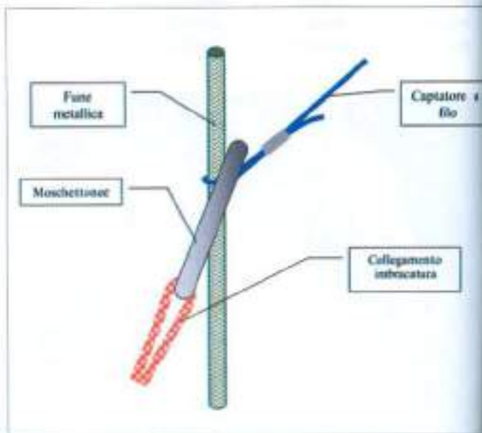
Fig. 5 - Captatore a filo
