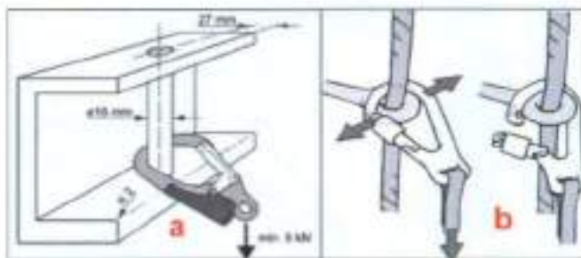
Fig. 3.a - La prova a flessione del moschettoni tipo K (da ferrata), prescritta dalla UIAA.
